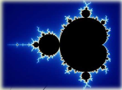
Mandelbrot halmaz
