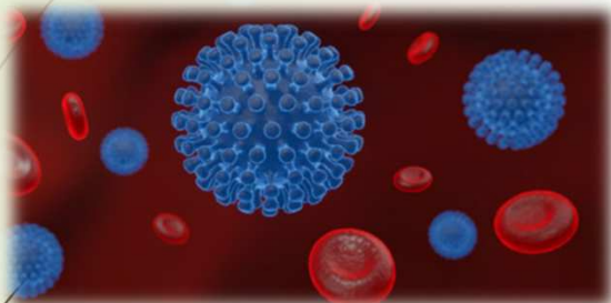
COVID vírus
